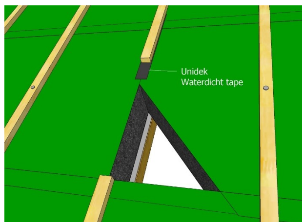
Figuur 5 - Detail verticale stootnaad
