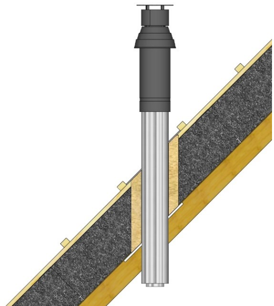
Figuur 7 - Detail sparring mantelbuis
