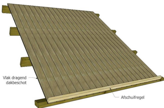
Figuur 3 - Afschuifregel op vlak dragend dakbeschot
