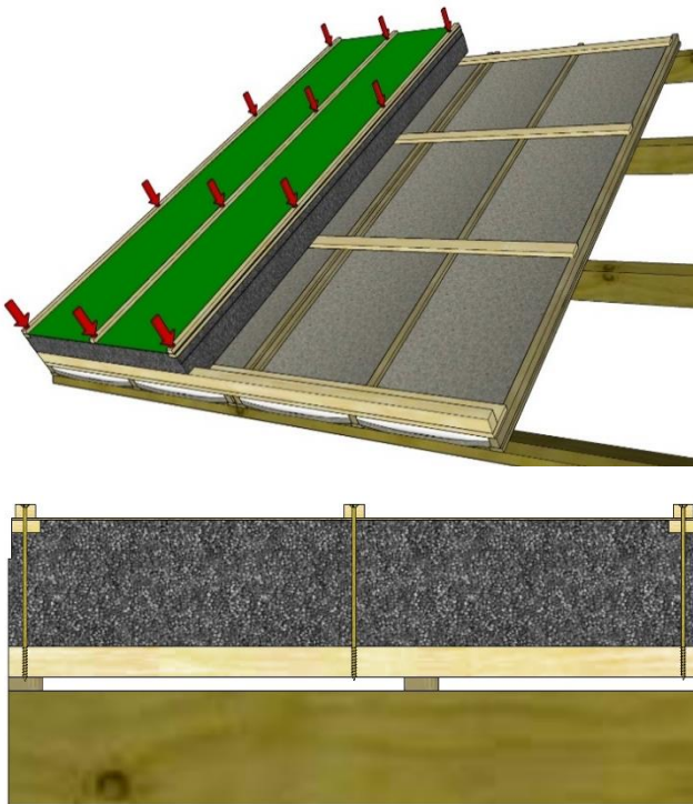
Figuur 8 - Bevestigingspunten
