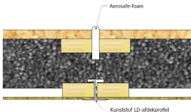
Figuur 5 - Detail Aerosafe-foam en Kunststof LD-afdekprofiel
