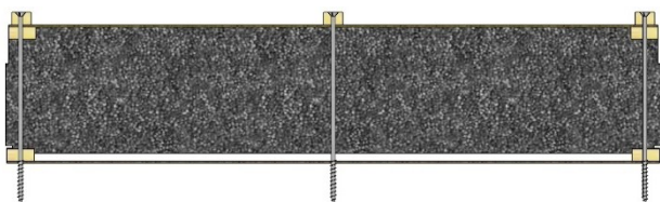
Figuur 3 - Detail bevestiging Unidek Aero Bio
