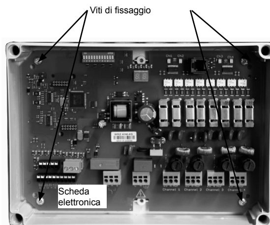
Fig.: WRZ 40M-4G con scheda elettronica
