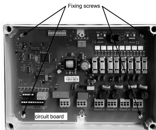
Fig.: WRZ 40M-4G with circuit board
