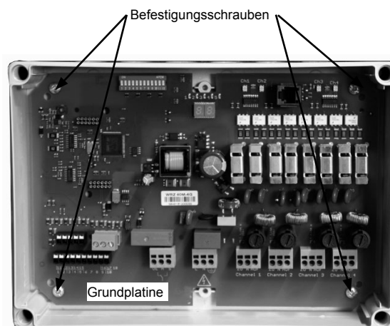
Abb.: WRZ 40M-4G mit Grundplatte
