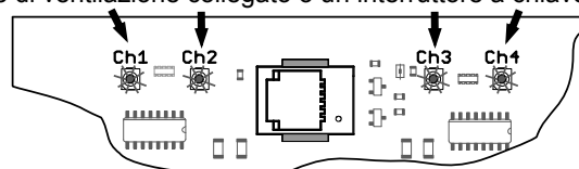
Fig.: LED dei gruppi motore collegati da Ch1 a Ch4
