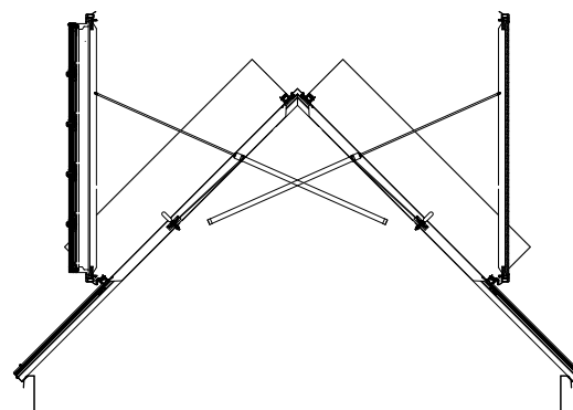
Doppelklappensystem, AirFlip (links) und FlatFlap (rechts) – Entrauchung position
