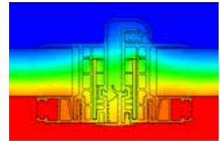
Isothermenverlauf AirFlip Lamellen- stoßbereich SLB im Schnitt
