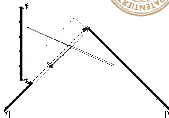
AirFlip Einzelklappensystem – Entrauchung position
