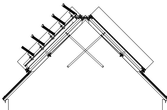
Doppelklappensystem, AirFlip (links) in Lüftung position 1) und FlatFlap (rechts)
