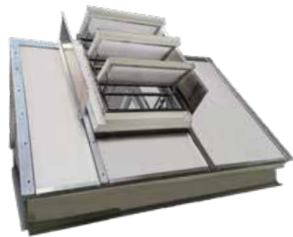
AirFlip Einzelklappensystem – Lüftungsposition
