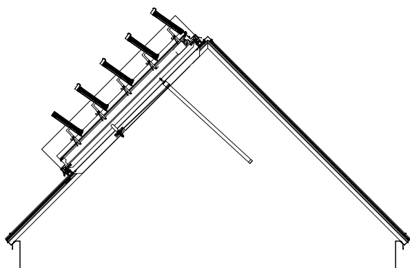
AirFlip Einzelklappensystem – Lüftung position
